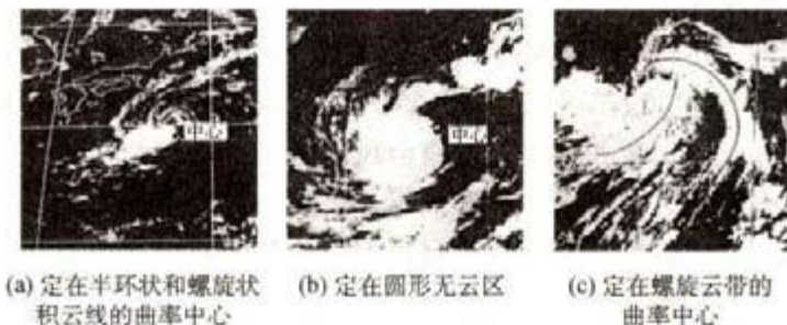
图 3.18 台风中心位于密蔽云区外部时（无眼）的卫星云图典型图例
