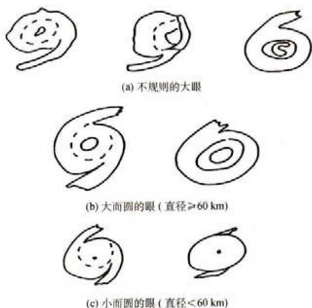
图 3.13 台风眼种类的示意图
