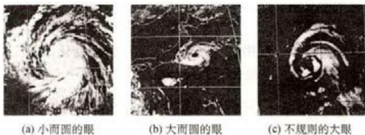
图 3.16 具有不同特征台风眼的卫星云图
