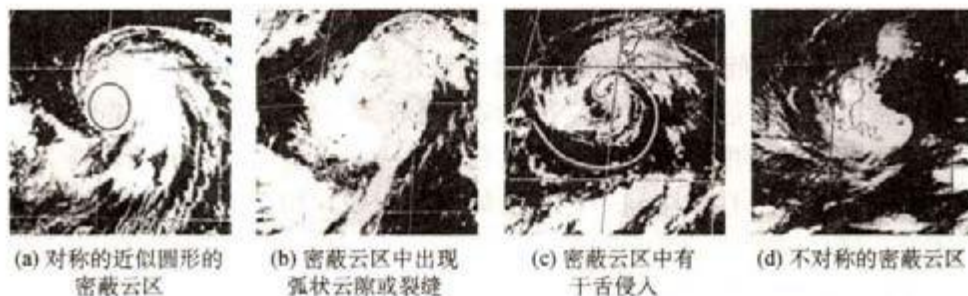
图 3.17 台风中心位于密蔽云区内部时（无眼）的卫星云图典型图例
