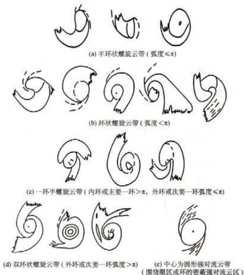
图 3.15 各种螺旋云带示意图
